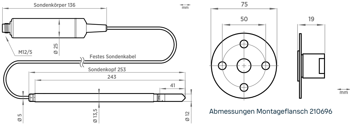
Abmessungen der HMP5
