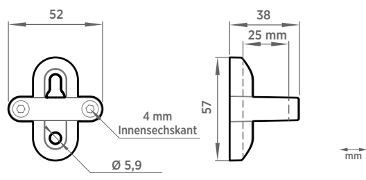
Abmessungen des Sondenhalters ASM213582
