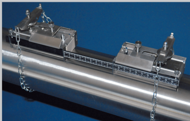
Messwandler-Befestigung
